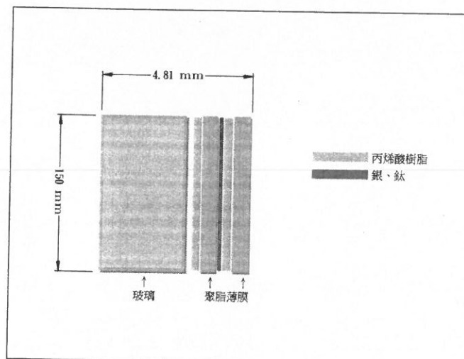
剖面圖
